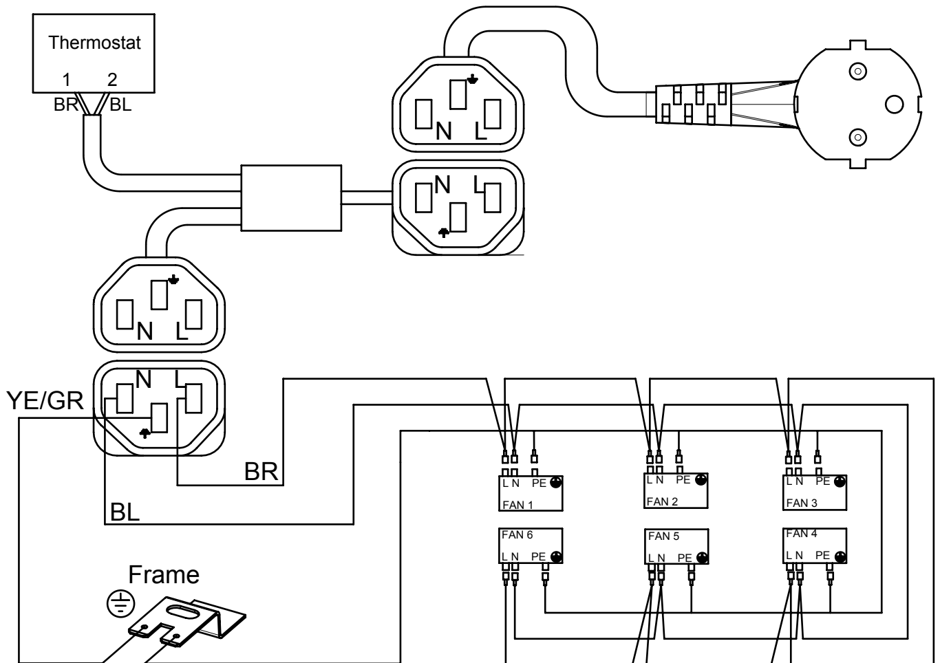
Verdrahtungsplan / Wiring diagram / Plan de câblage
